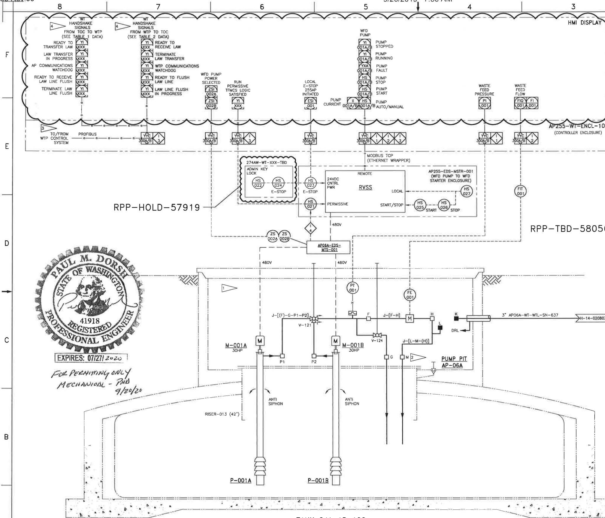
TANK 241-AP-106 SCALE: NONE
